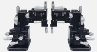
六轴调整架 FT2300B
