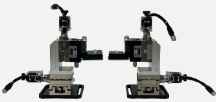
半自动六轴调整架 FTSA6100
